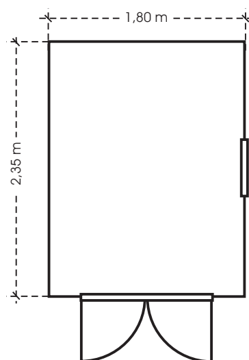
Postvundamendi näidisskeem
